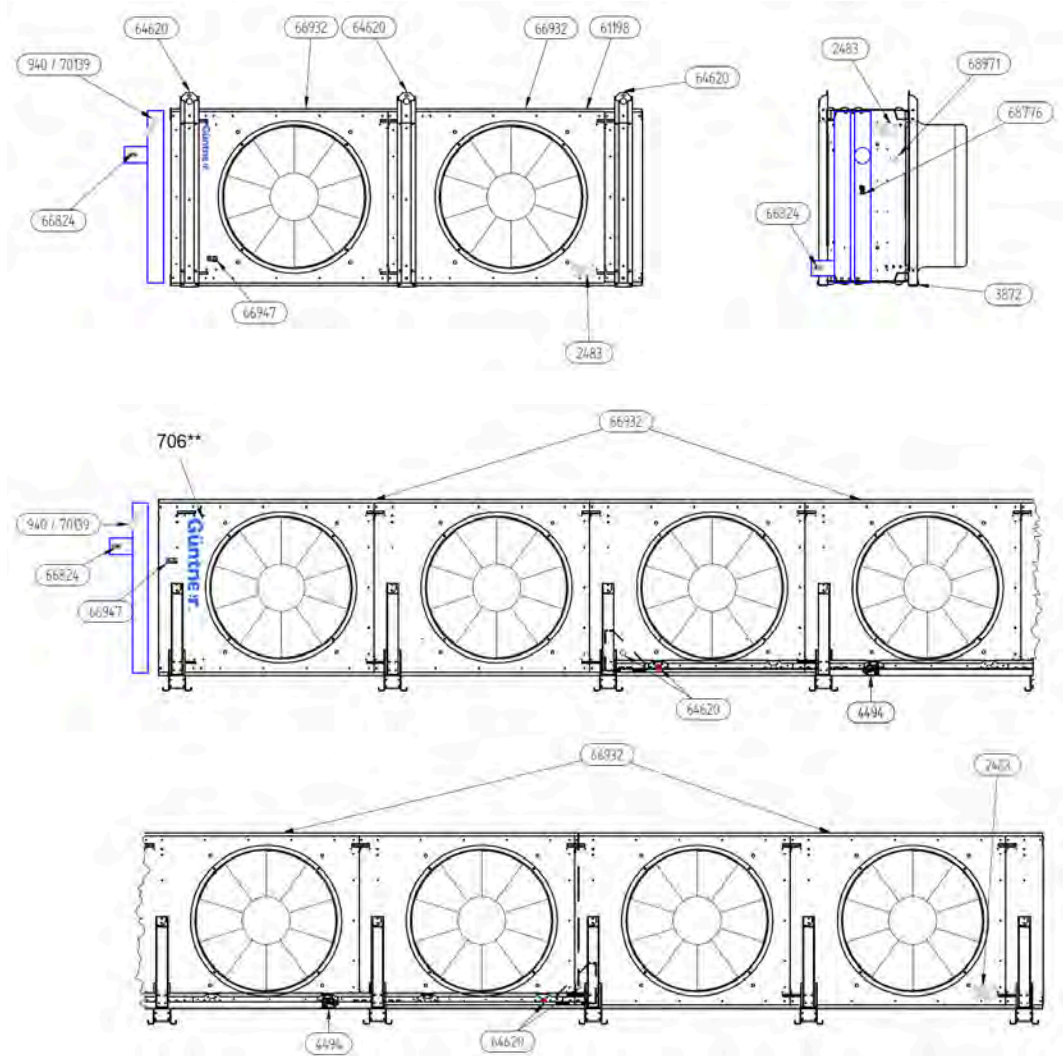
Vues du type I
