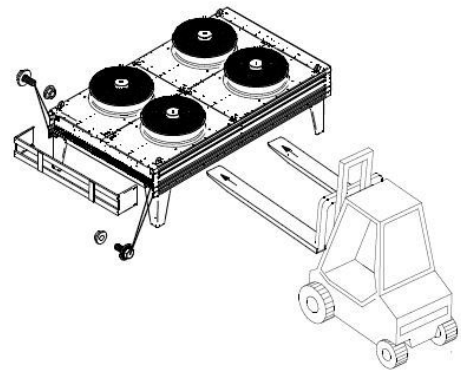
Déballage d'appareils horizontaux
