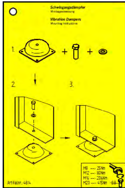
4814 – Mention sur les amortisseurs de vibrations (pour type I)
