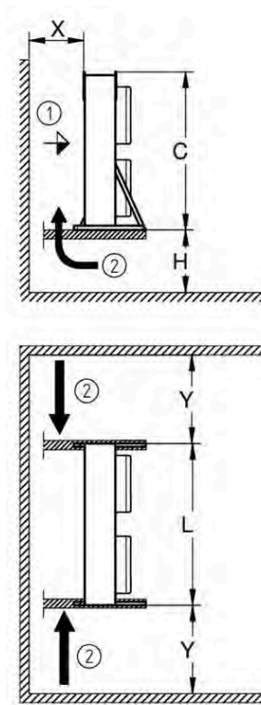
Montage mural ; Vue de côté (en haut) et vue de dessus (en bas)
