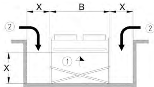
Installation dans un renforcement
