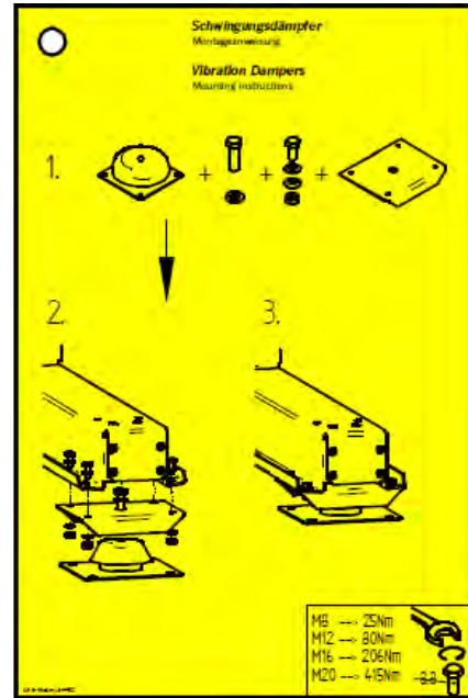
4492 – Mention sur les amortisseurs de vibrations (pour types II et III)
