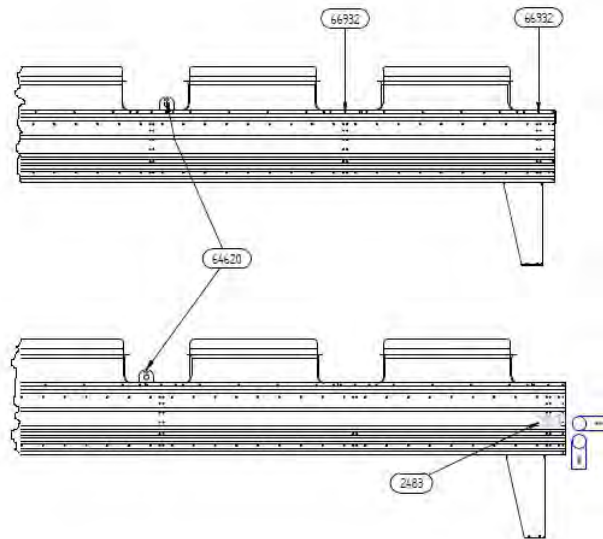
Vues séparées A (en haut) et B (en bas) – côté droit
