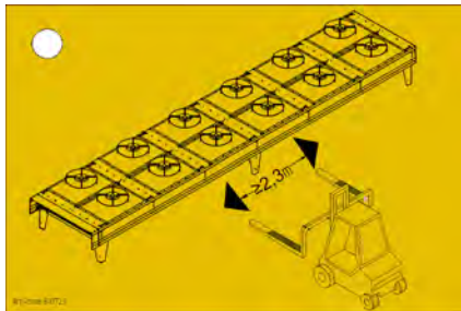
61072.1 – Plaque d'utilisation pour chariot de manutention à fourche pour appareils à deux rangées
