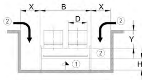
Installation dans un renforcement – buses de sortie d'air
