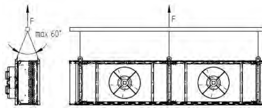
Illustration des opérations de transport pour Vertical VARIO de type I
