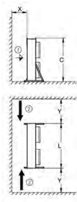
Installation au sol ; Vue de côté (en haut) et vue de dessus (en bas)
