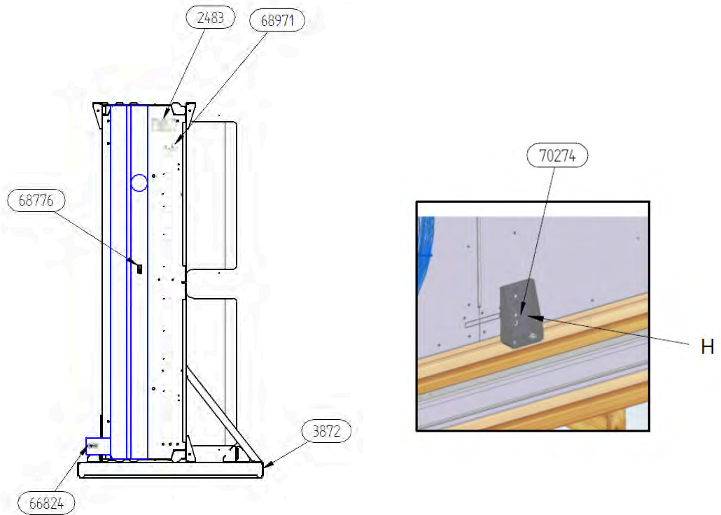
H – Support pour appareils Flat pour le transport vertical
